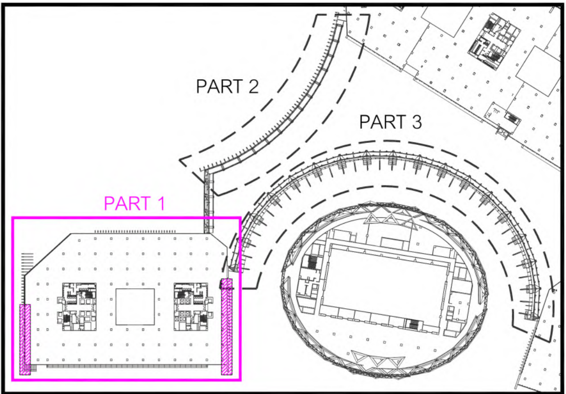
อาคารทิศตะวันตก : ผังพื้นที่ติดตั้งดวงโคมชั้น 1 (PART1) มาตราส่วน 1 : 200 @ A1
