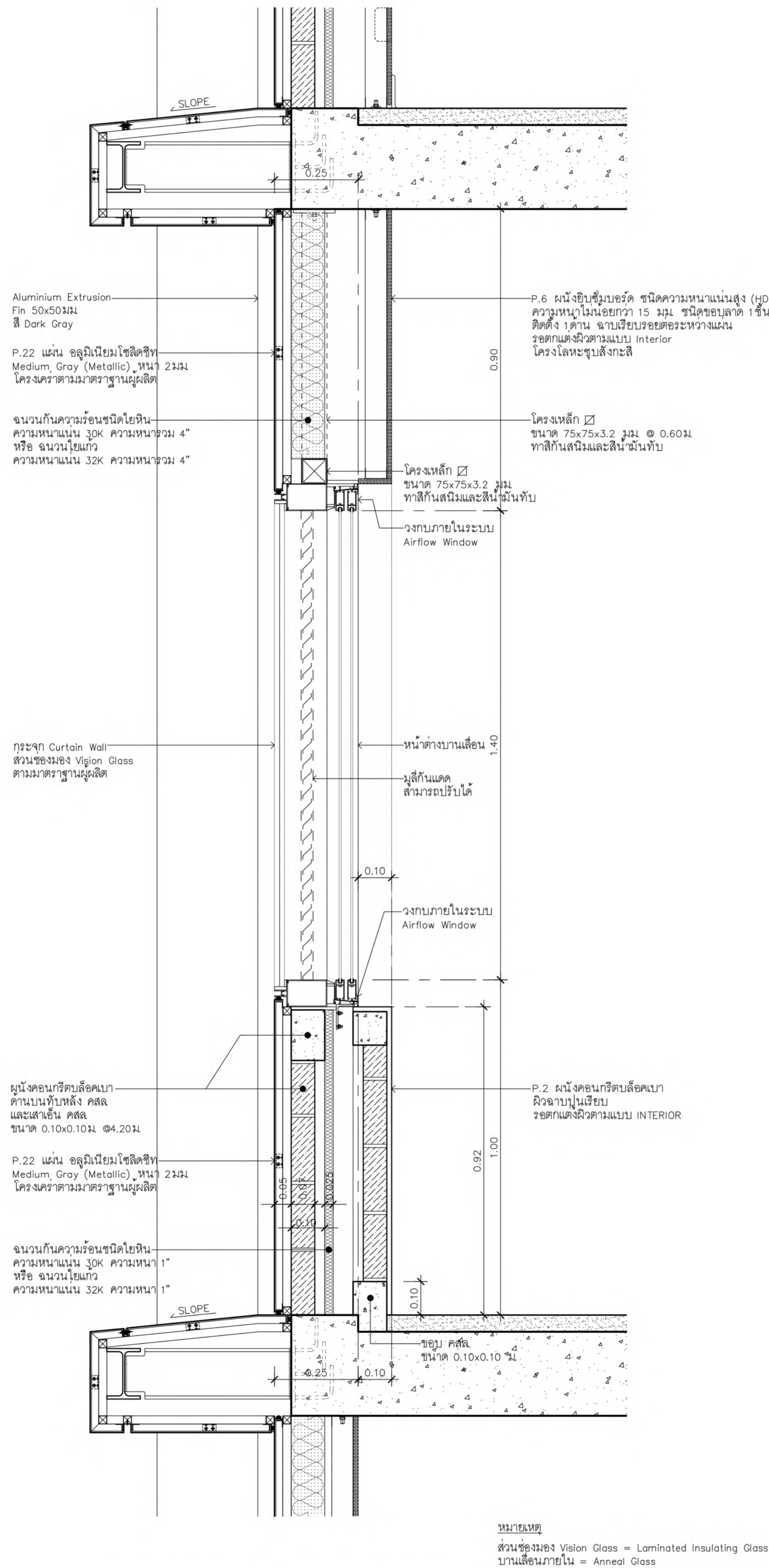
แบบขยายผนัง CURTAIN WALL 3.1 มาตราส่วน 1:10
