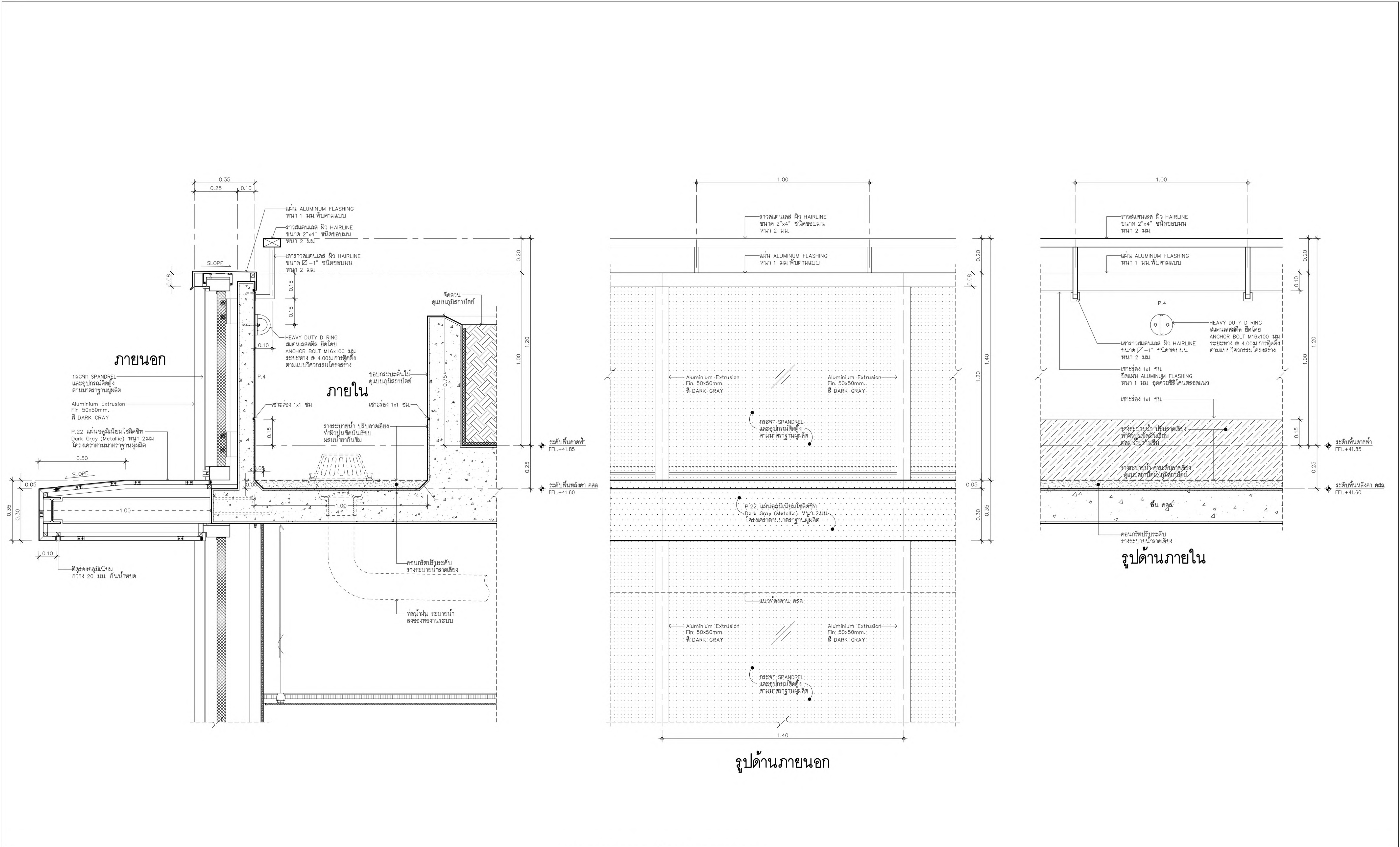
แบบขยาย รากันตกภายนอก 3 มาตราส่วน 1:10
