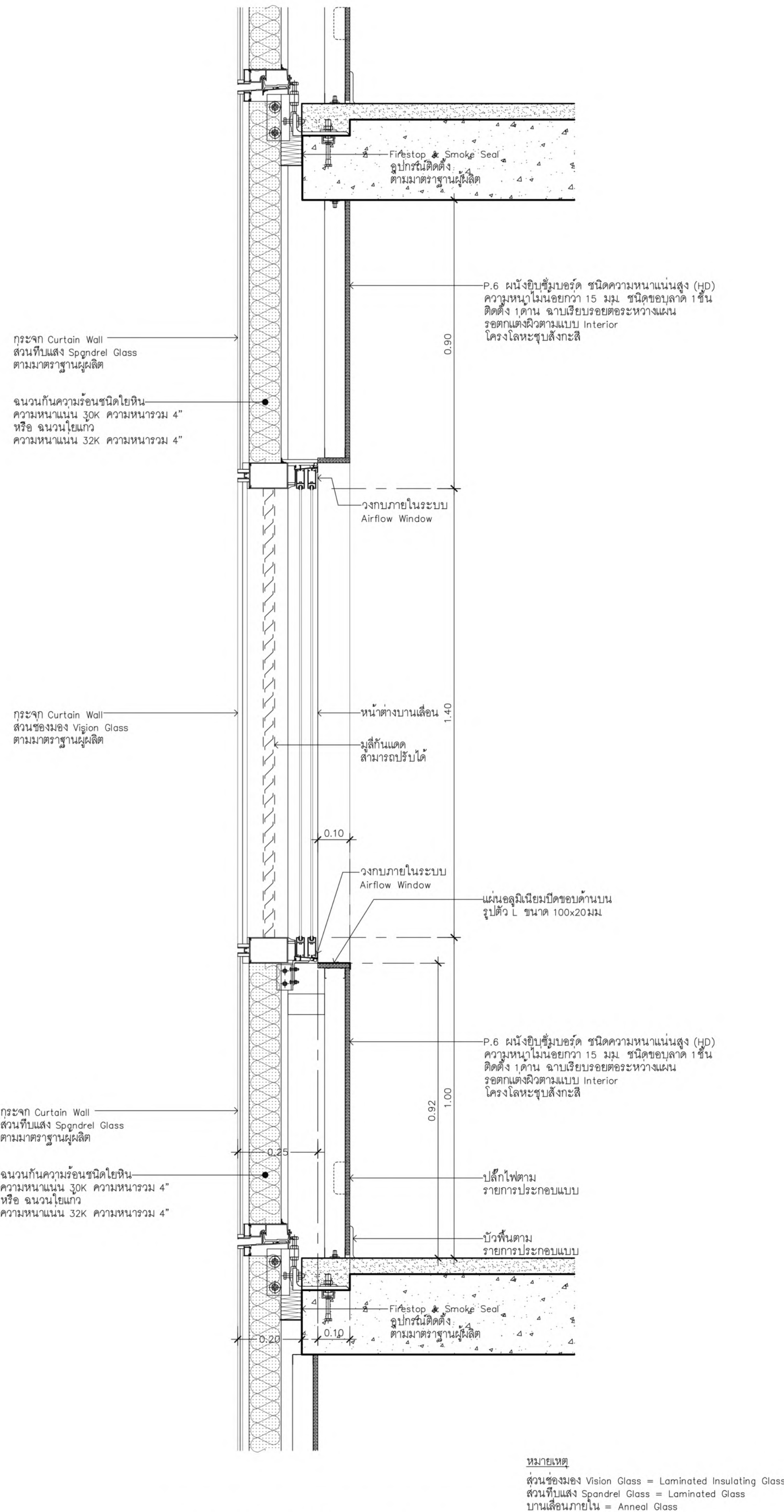
แบบขยายผนัง CURTAIN WALL 5 มาตราส่วน 1:10
