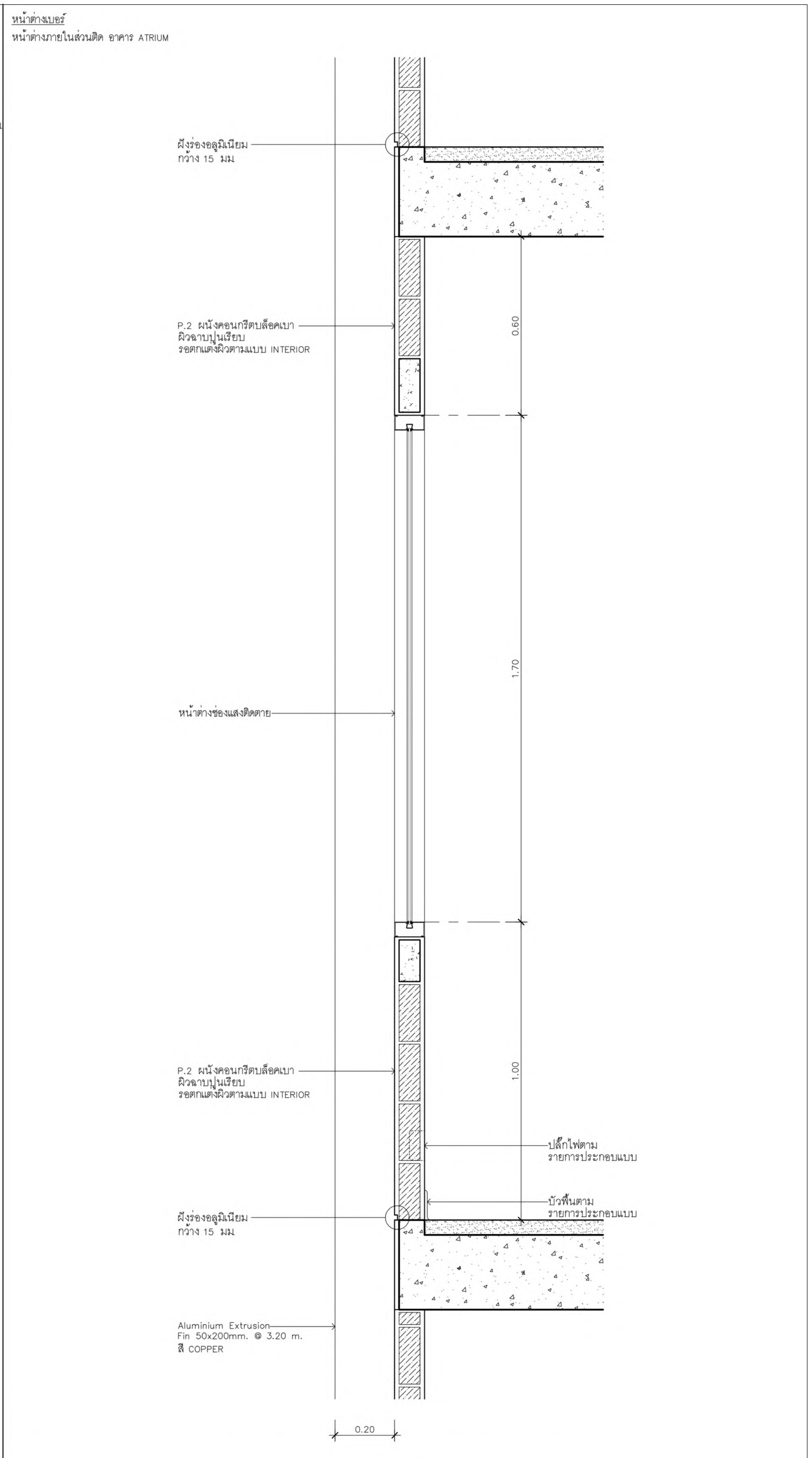
แบบขยายผนัง CURTAIN WALL 7 มาตราส่วน 1:10
