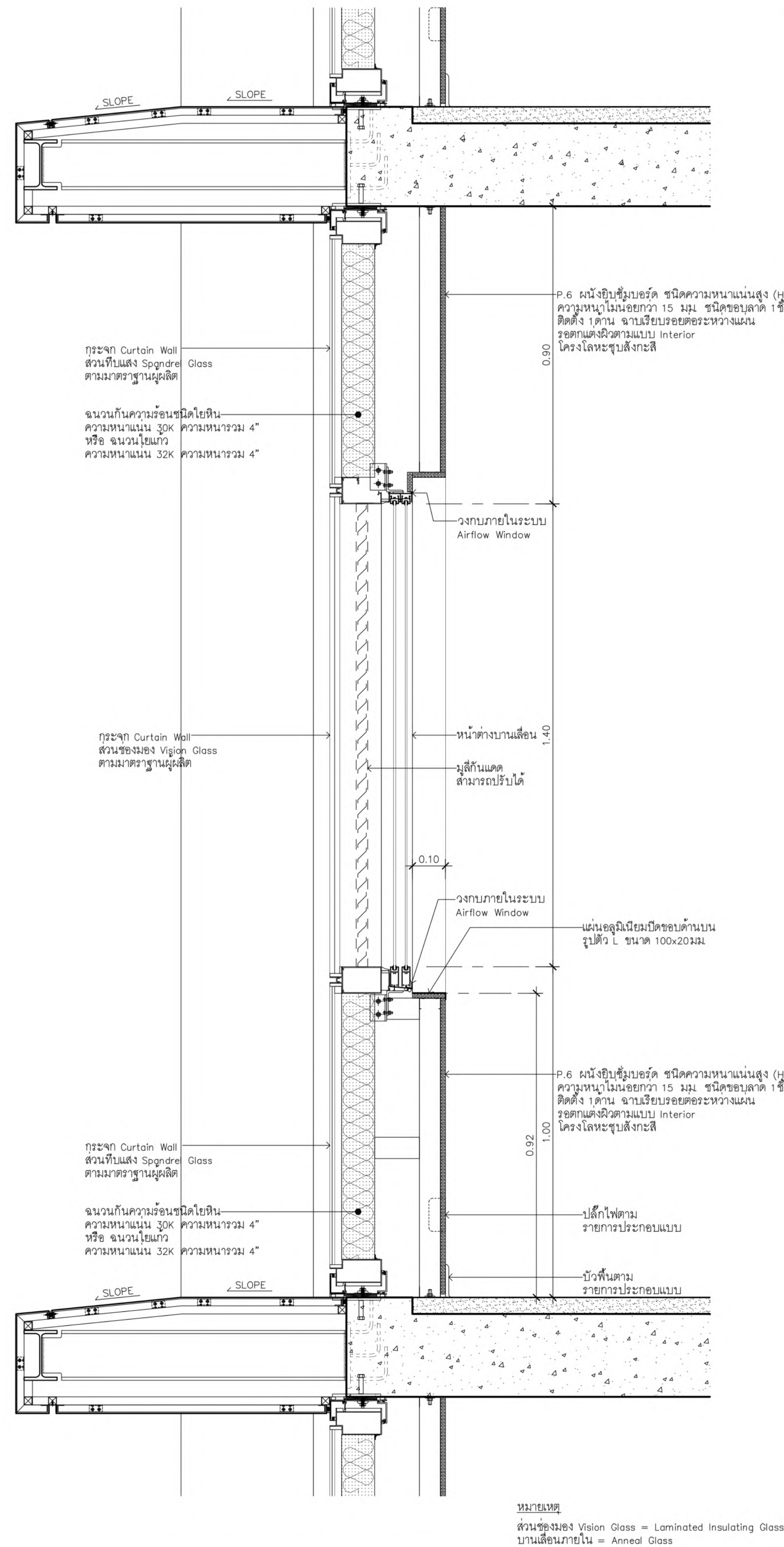
แบบขยายผนัง CURTAIN WALL 4 มาตราส่วน 1:10
